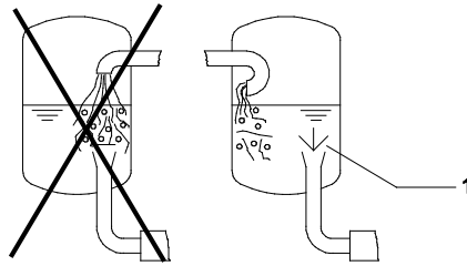
Afb. 9: Positie tankinlaat/tankuitloop
