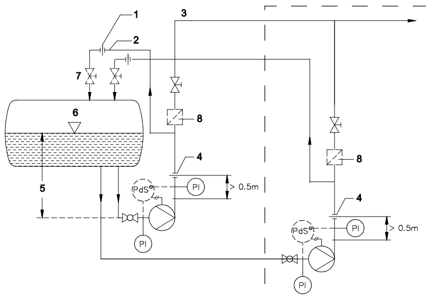
Afb. 13: Automatische ontgassing (enkele pomp - parallelpompen)
