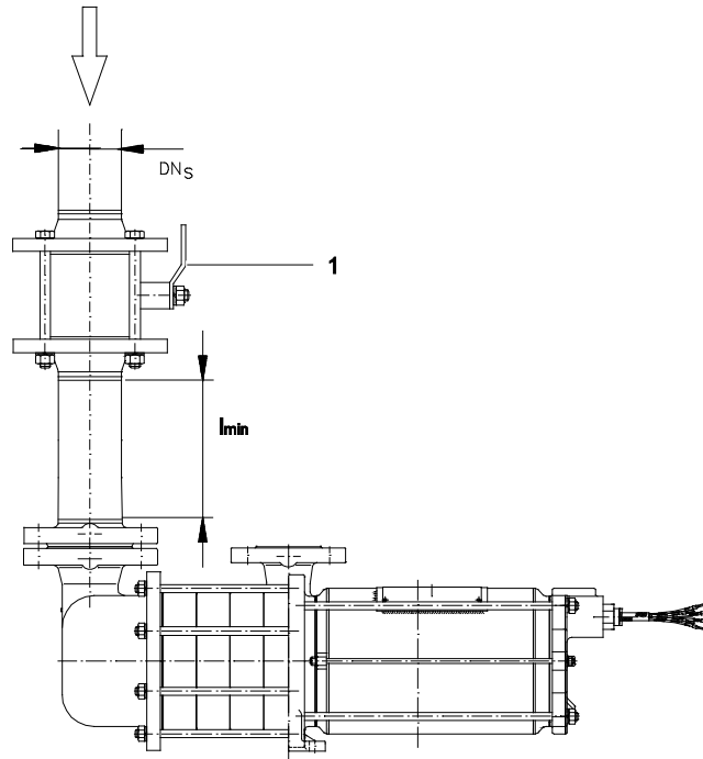
Afb. 7: Toevoerleiding
